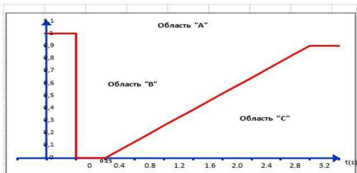
Рисунок 1. Условия устойчивой работы ВЭС определены характеристикой «напряжение-время».
