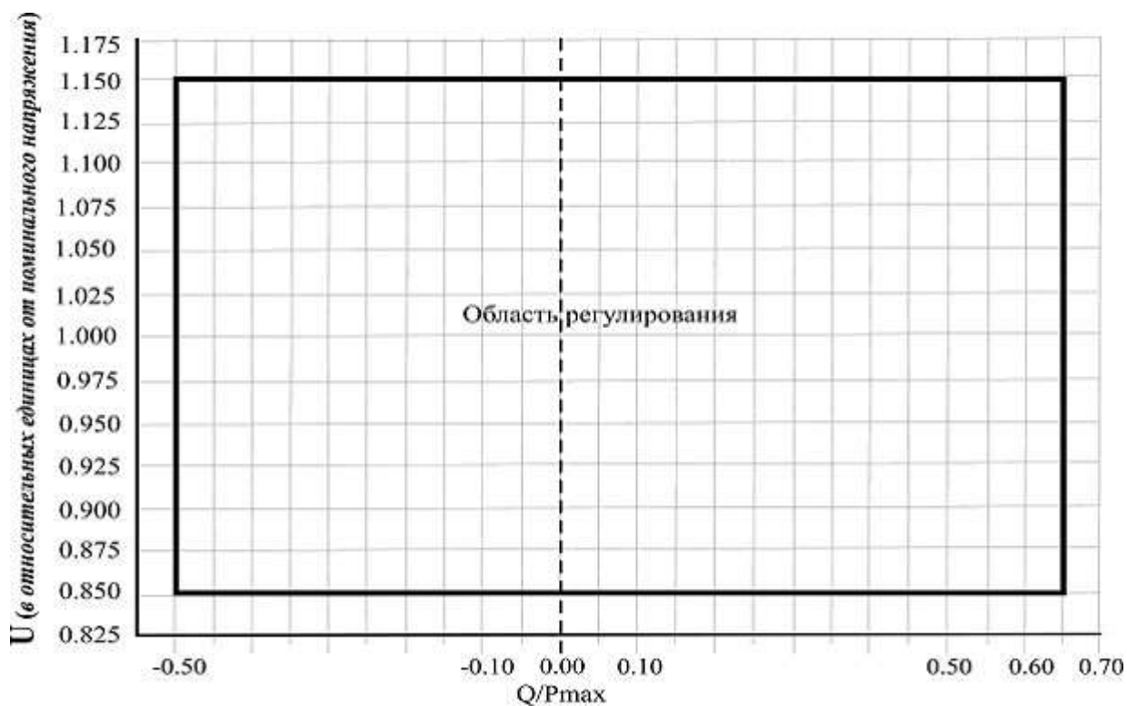
Рисунок 3. Зависимость регулировочного диапазона по реактивной мощности СЭС от фактического напряжения в точке подключения.
